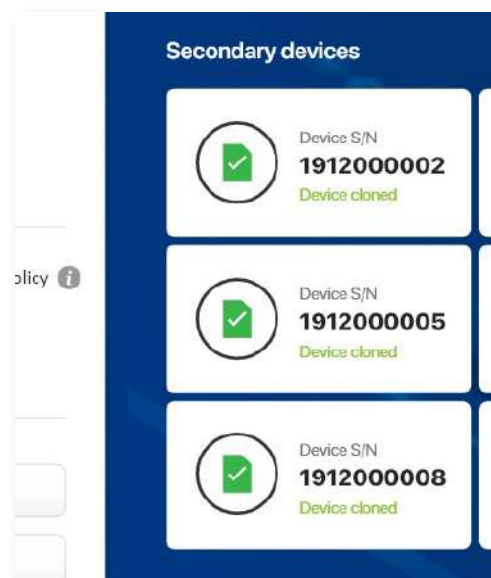
Bild 11: Klonen abgeschlossen
